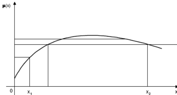
Слика 1. Konveksni fyzyy skup Извор: S.Џурић, 2005., str. 17.
